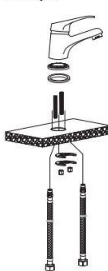
Схема 2 2 штифта
