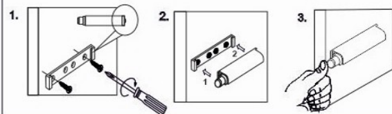
Схема установки механизма Push to open
