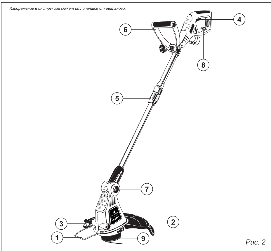
Рис.2. Расположение основных элементов электротриммера:
