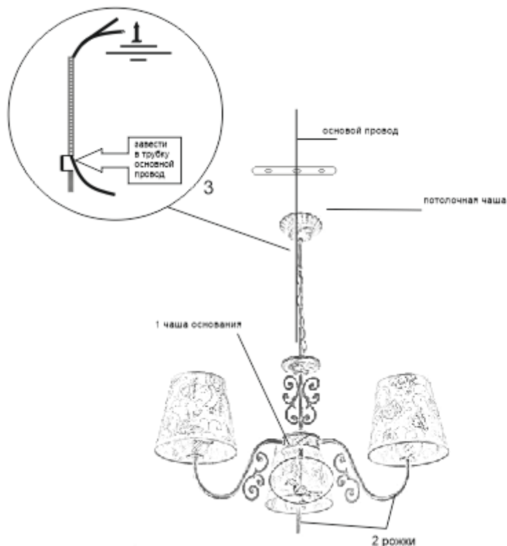
Рис.1 Сборка светильника
