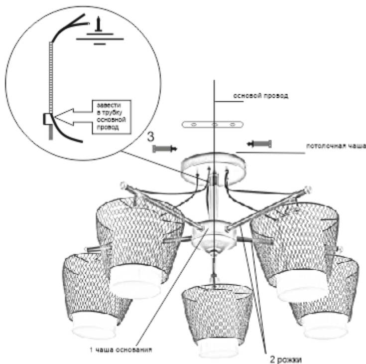
Рис.1 Сборка светильника
