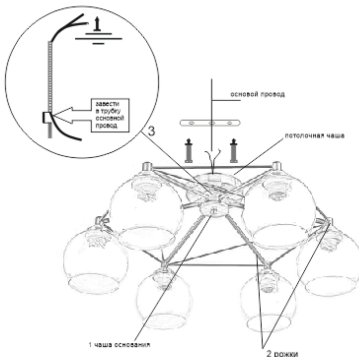
Рис.1 Сборка светильника
