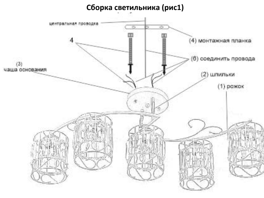
Рис.1 Сборка светильника
