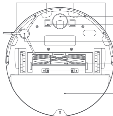
Rotella omnidirezionale Contatti di ricarica Sensore di movimento Spazzola laterale Rotelle principali Spazzola principale Fermi per protezione spazzola Serbatoio dell'acqua
