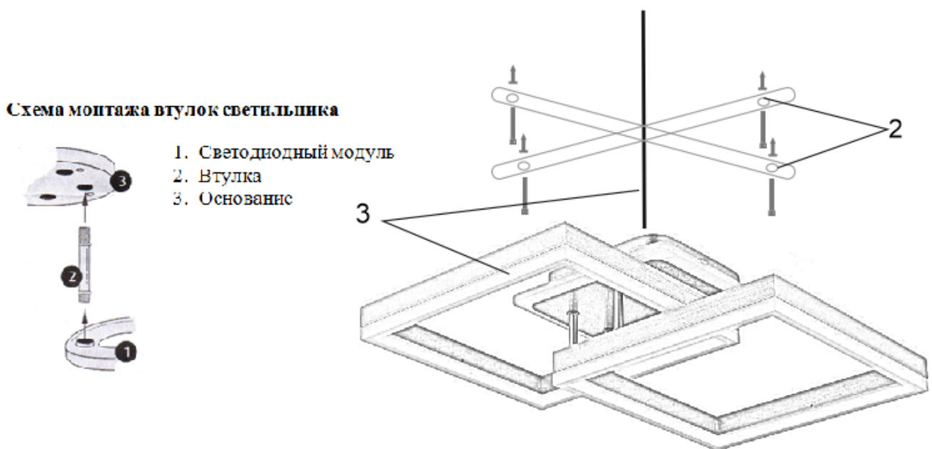
Сборка светильника (рис1)
