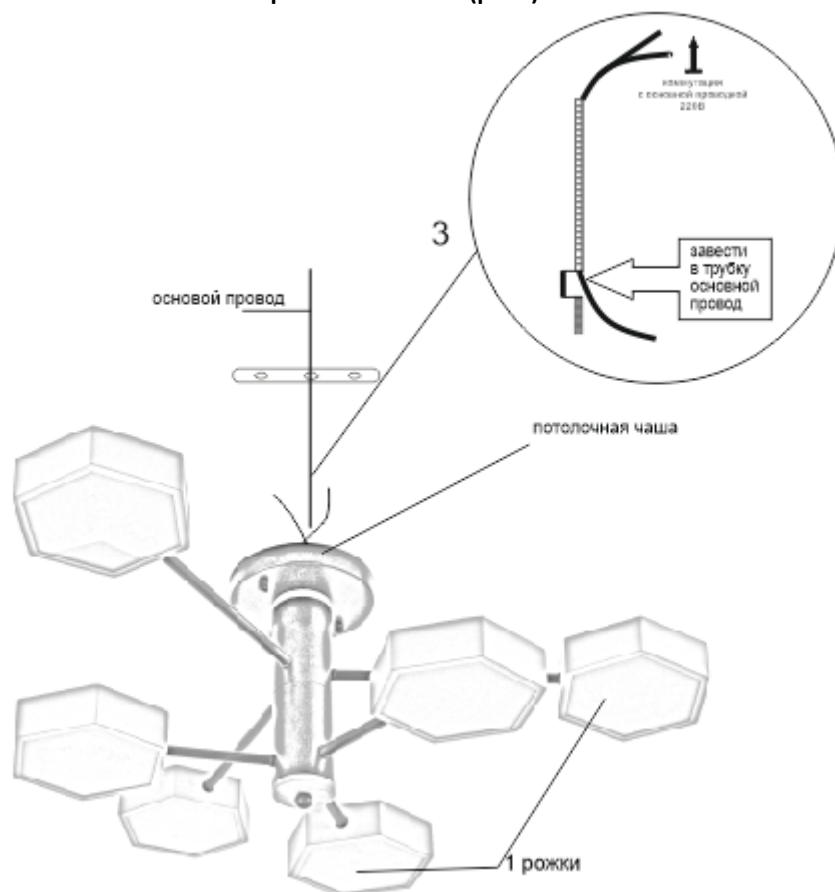
Сборка светильника (рис1)
