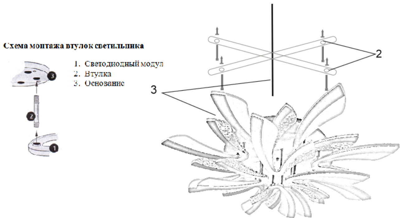
Сборка светильника (рис1)
