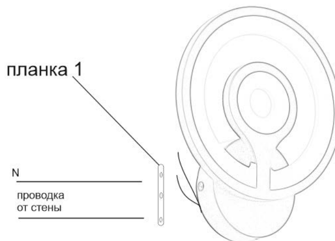
Рис.1 Сборка светильника
