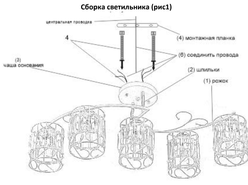
Рис.1 Сборка светильника
