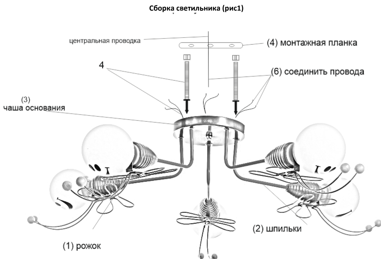
Рис.1 Сборка светильника
