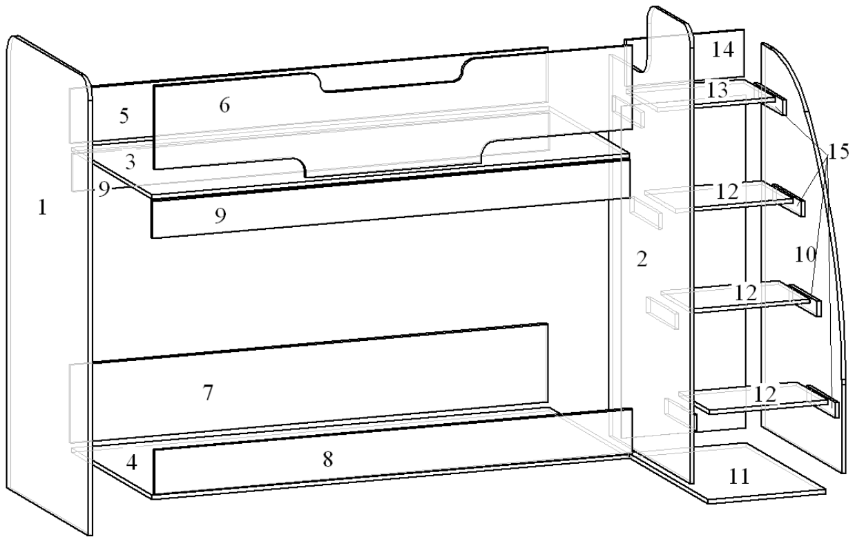
Сборка ящика кровати.
