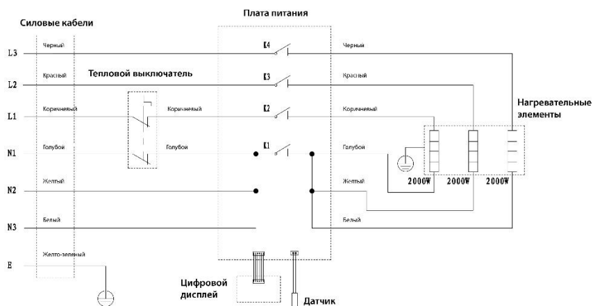
Рисунок 3. Электрическая схема подключения
