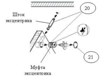
Рис.2 Установка эксцентриковой стяжки
