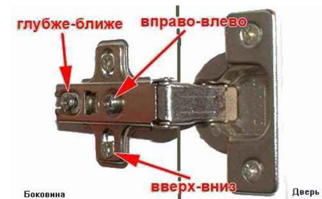
Рис.5 Крепление и регулировка петель
