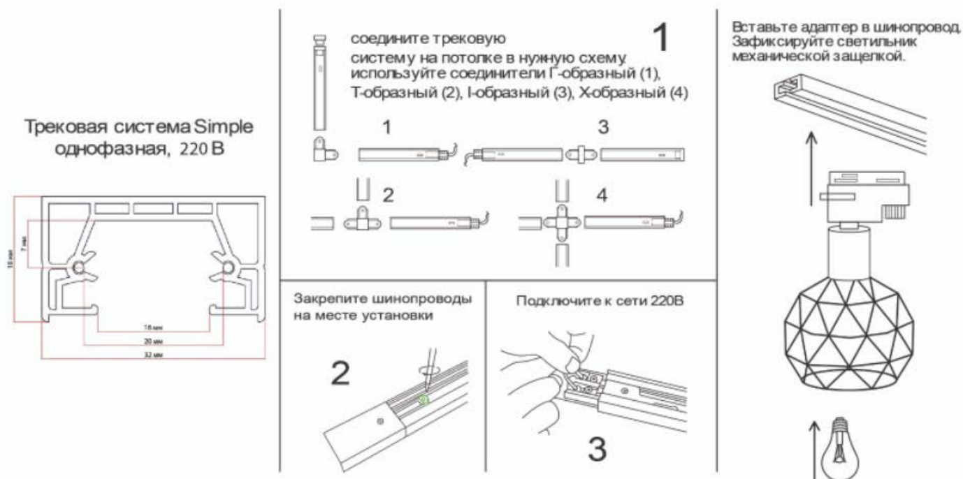
Рис.1 Сборка светильника
