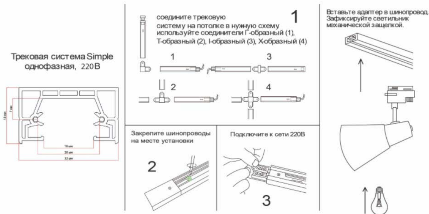
Рис.1 Сборка светильника
