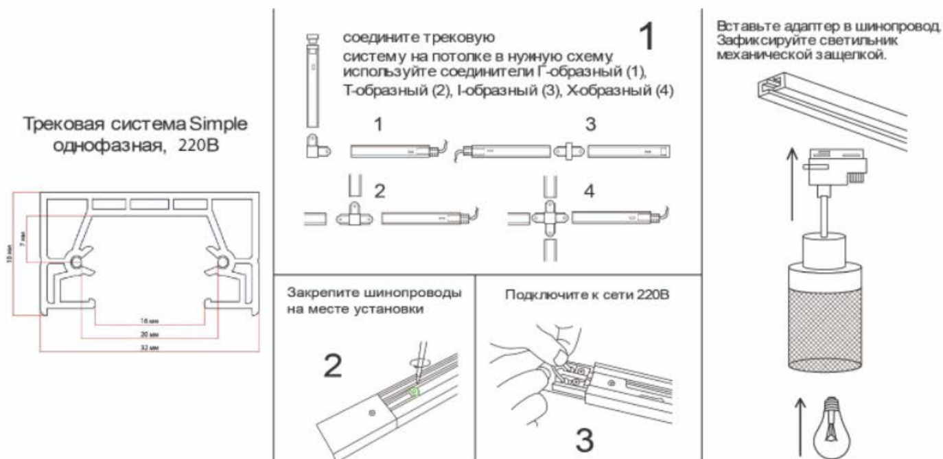
Рис.1 Сборка светильника
