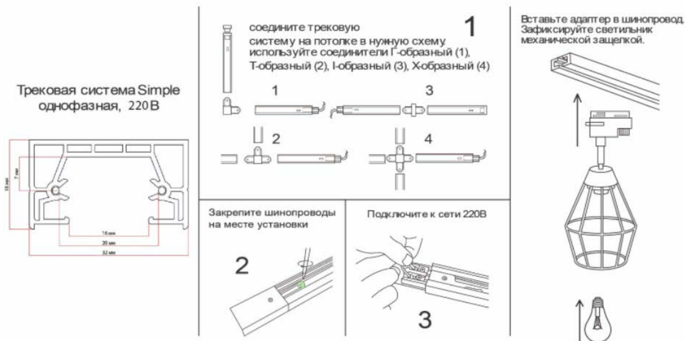
Рис.1 Сборка светильника
