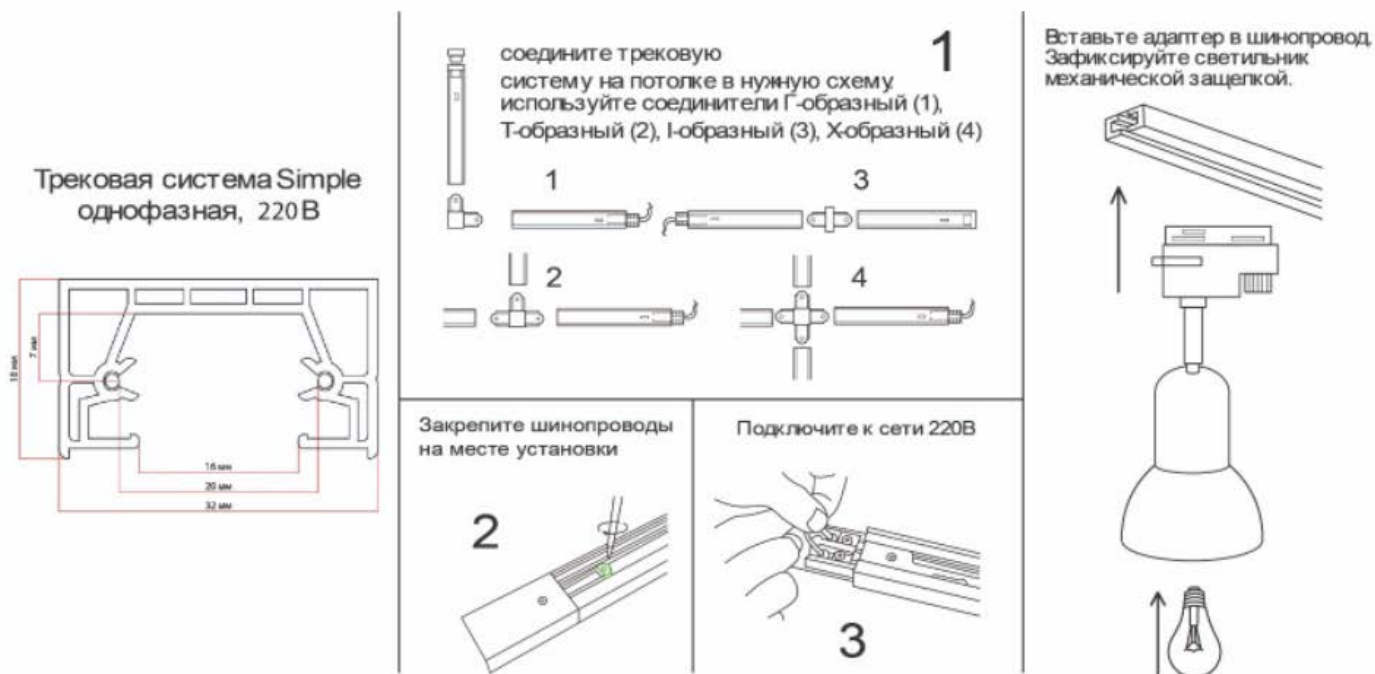
Рис.1 Сборка светильника
