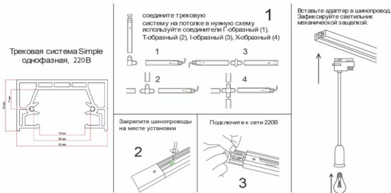
Рис.1 Сборка светильника
