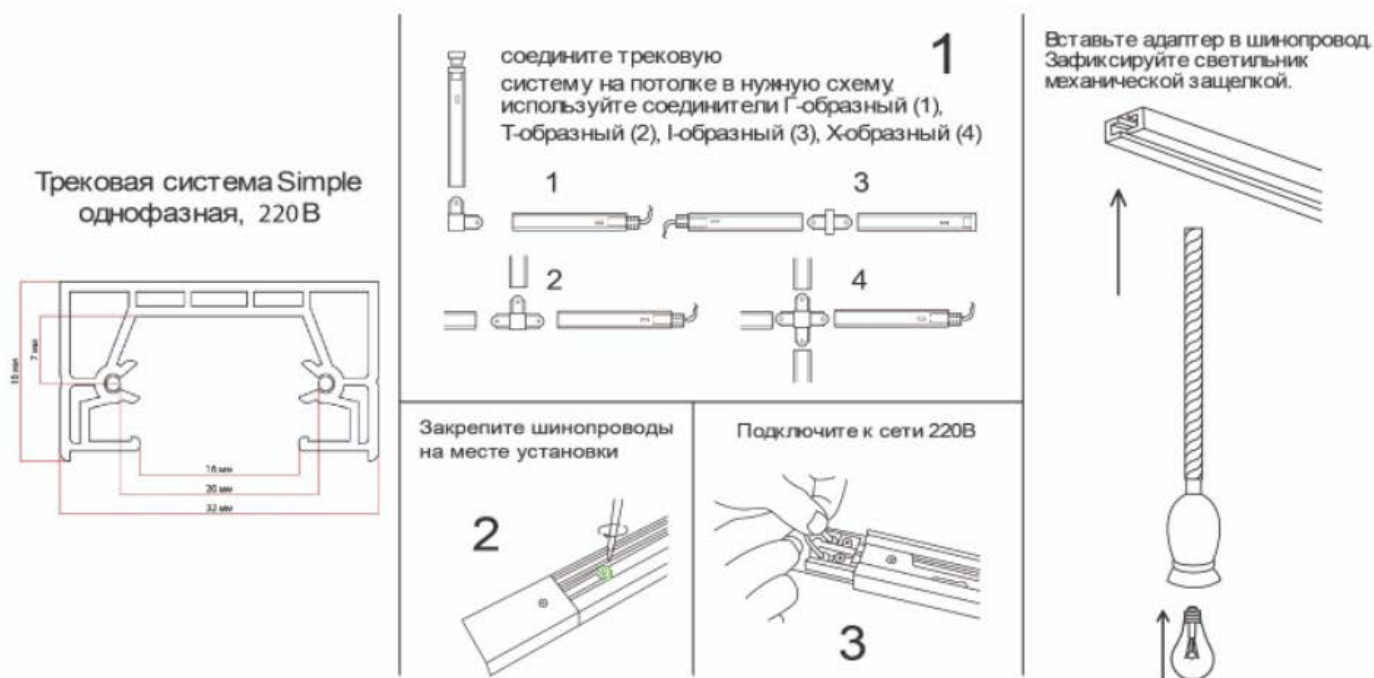
Рис.1 Сборка светильника
