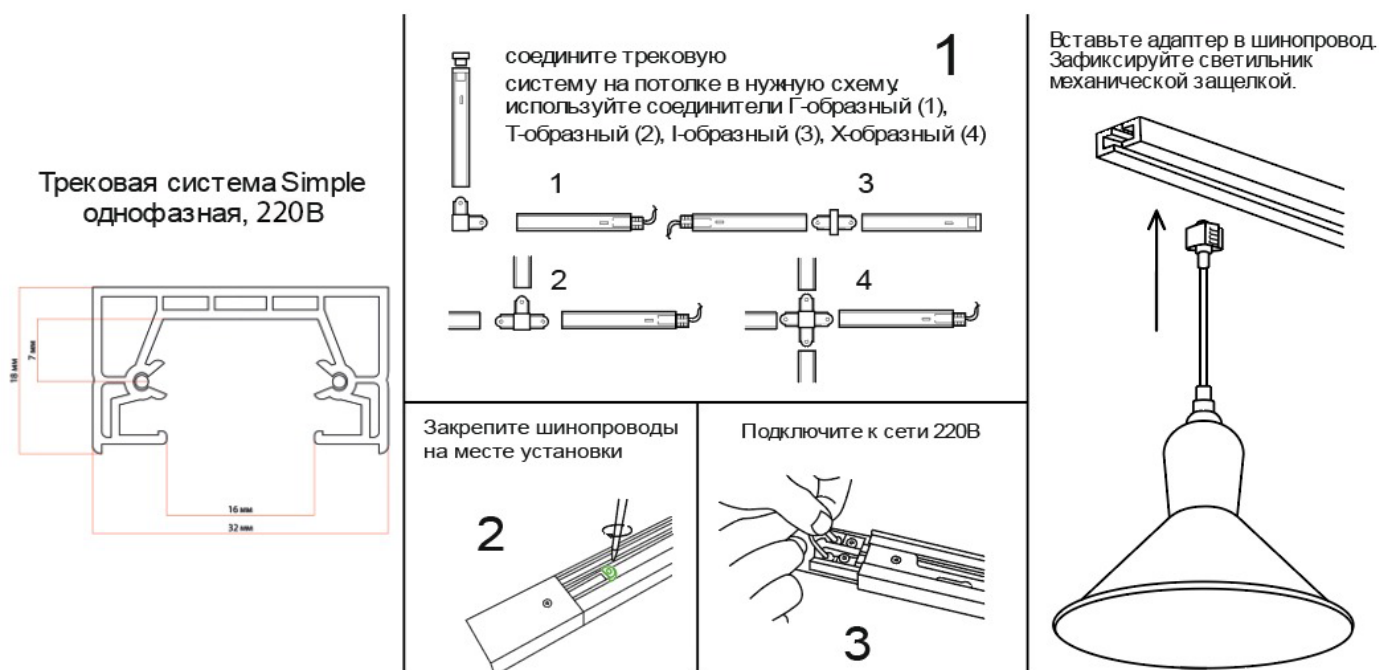
Рис.1 Сборка светильника
