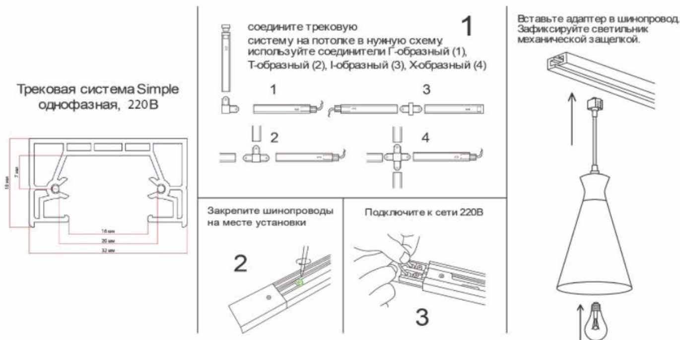
Рис.1 Сборка светильника
