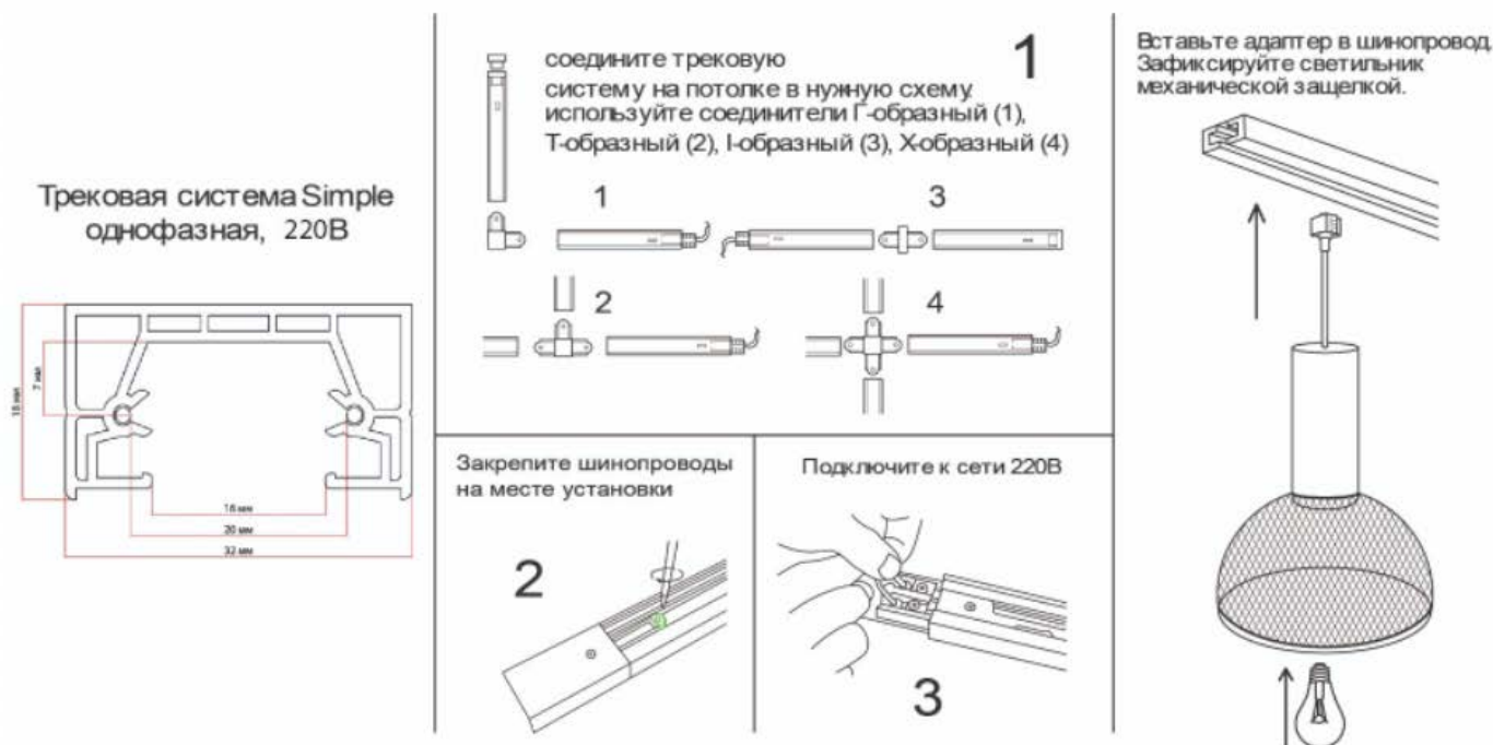
Рис.1 Сборка светильника
