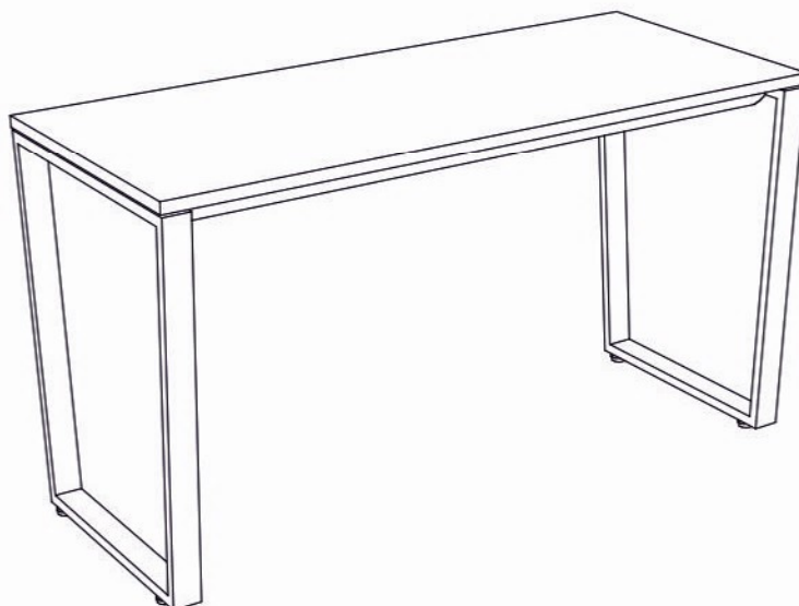
Алиса мод. 14 Стол универсальный Гринвич мод. 11 Стол универсальный Стол Флай артикул Ж.01.07.08.01 Размеры (ВхШхГ) 737x1340x590
