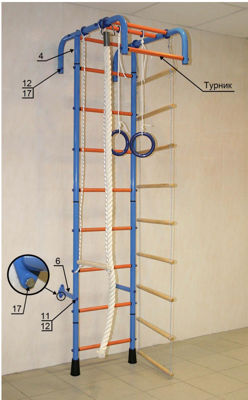
Рис.3. Вариант сборки ДСК-3-5 с креплением к стене
