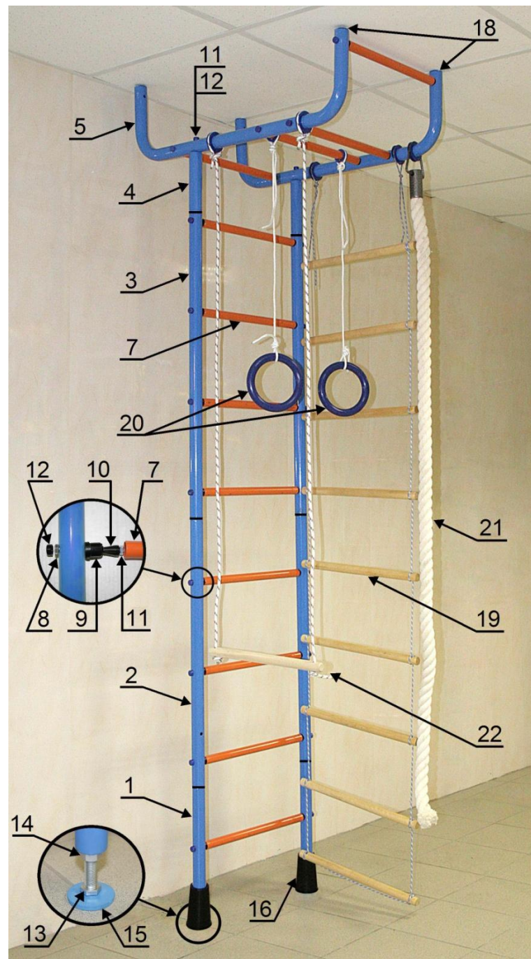
Рис.2. Вариант сборки ДСК-3-5 с креплением враспор между полом и потолком
