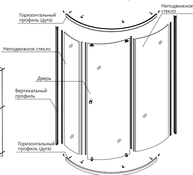
⚠ Ограждение Simple типовая сборка
