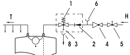
Montage unterhalb des Waschbeckens
