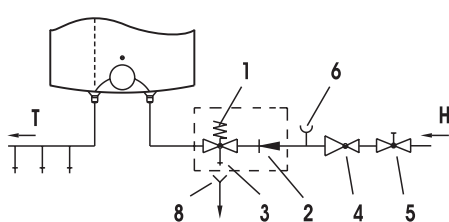
Варијанта иазад умиваоника
