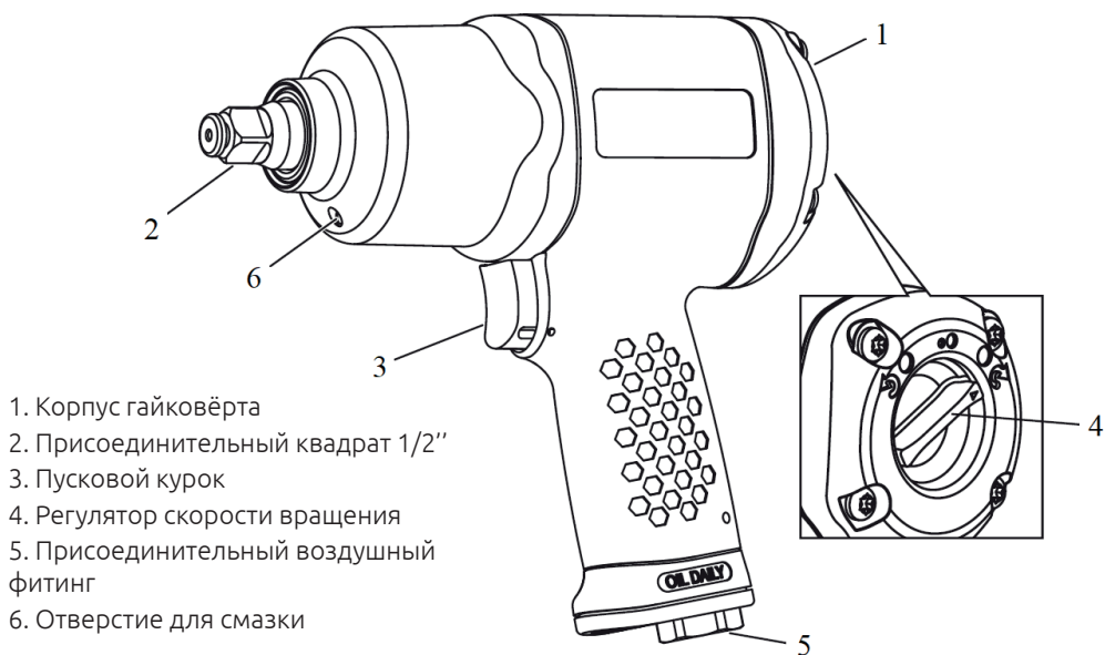
Рис. 1. Основные элементы пневматического гайковёрта «КВАЗАР»
