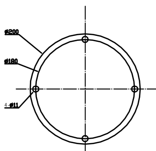
预埋件位置图
