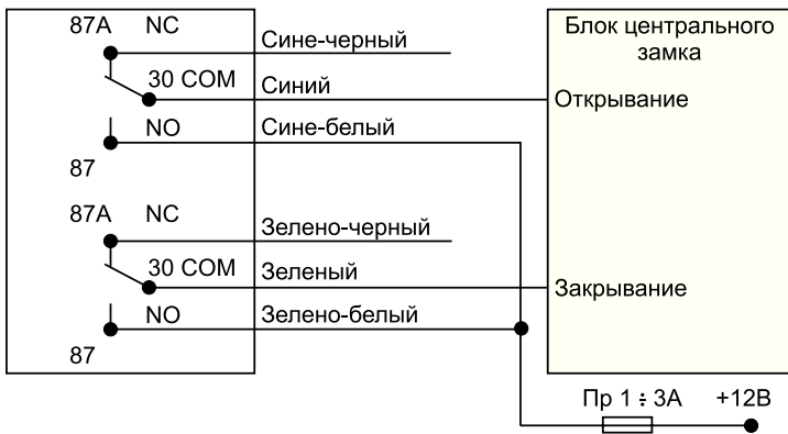
Управление Ц.З. положительными импульсами (время упр. 0.8 сек)
