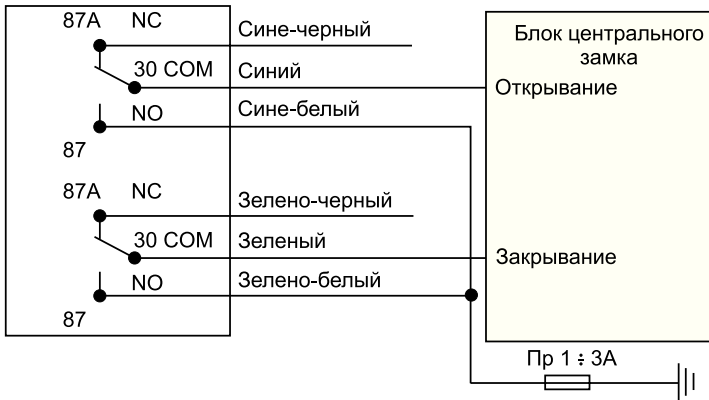
Управление Ц.З. отрицательными импульсами (время упр. 0.8 сек)
