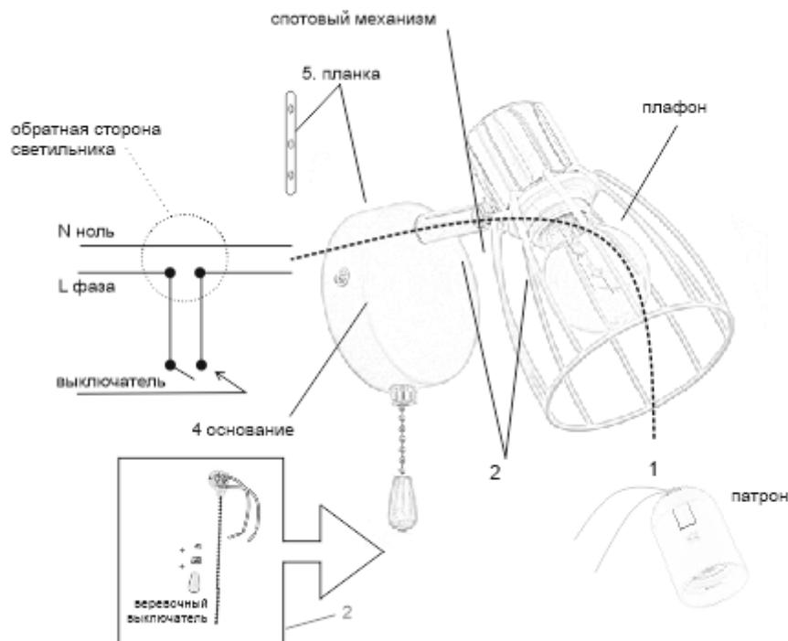
Рис.1 Сборка светильника
