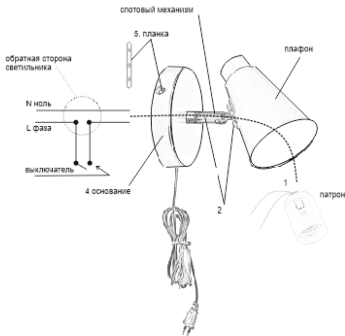
Рис.1 Сборка светильника
