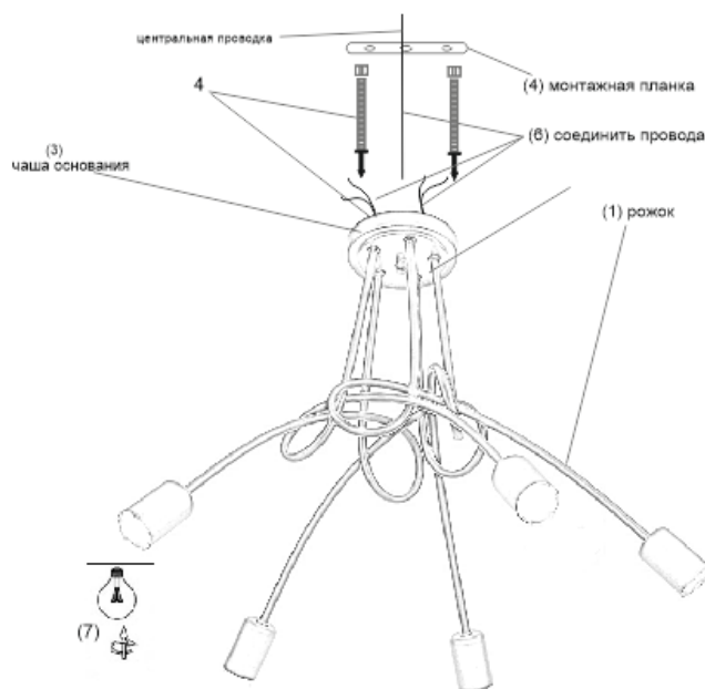
Рис.1 Сборка светильника
