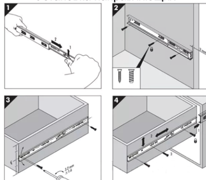
Установка направляющих
