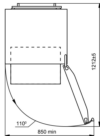
Figura 2 – Frigiderul (vedere de sus)
