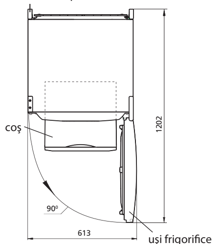
Figura 2 – Congelator (vedere de sus)
