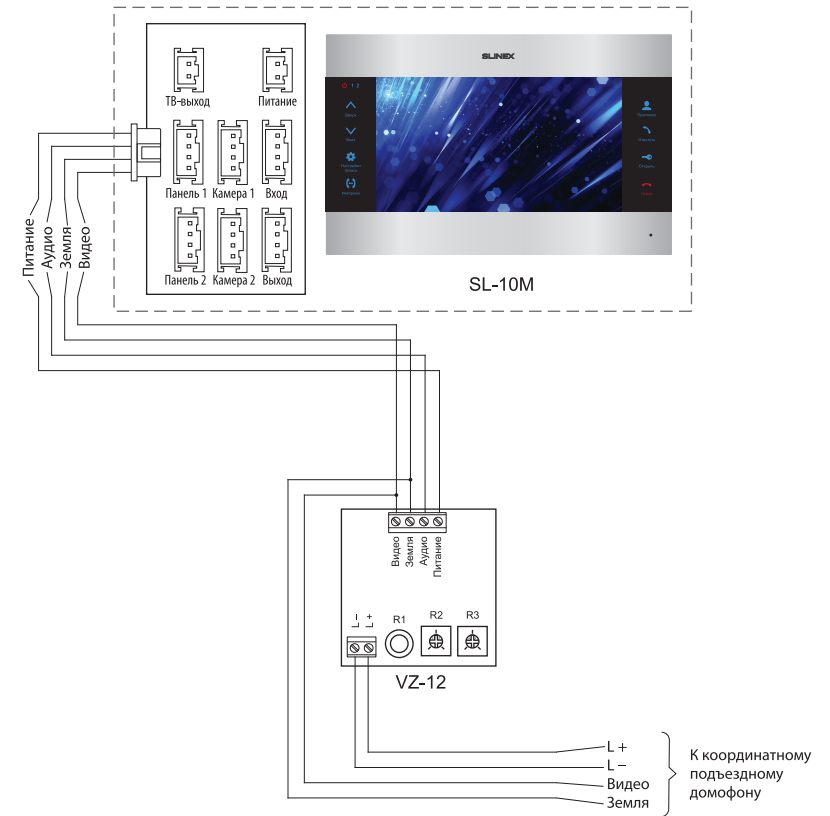
Схема подключения адаптера VZ-12
