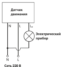
Рис. 1 Схема подключения
