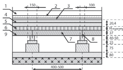
Рис. 18. Укладка напольного покрытия на старом дощатом полу: использование ГВЛ или фанеры
