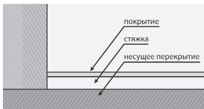
Рис. 13. Соединительная стяжка
