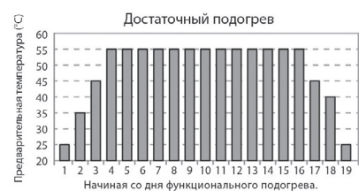
Рис. 16. Достаточный подогрев
