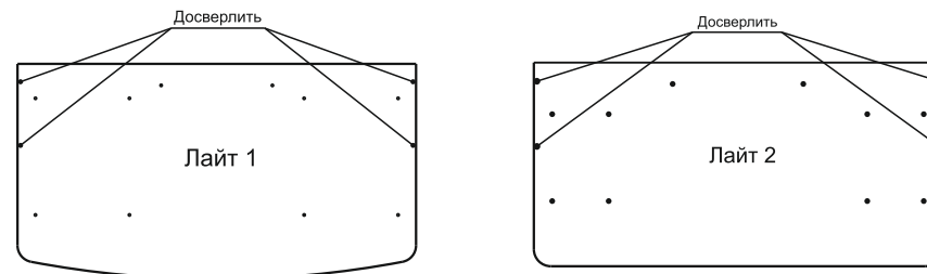
Схема 4. Досверливание отверстий (стол компьютерный 1200 «Лайт 1» и «Лайт 2»)
