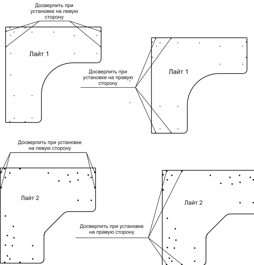
Схема 5. Досверливание отверстий (стол комп. угловой 1200 «Лайт 1» и «Лайт 2»)
