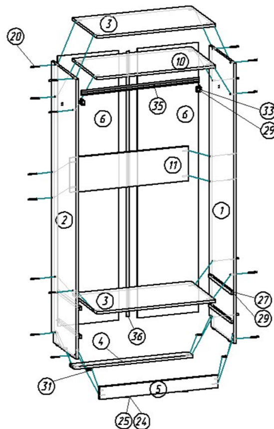
Рис.1 Сборка корпуса
