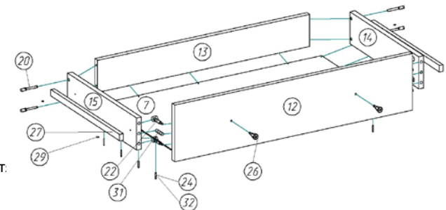
Рис.5 Сборка ящиков
