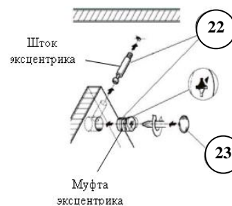
Рис.4 Установка эксцентриковой ст.
