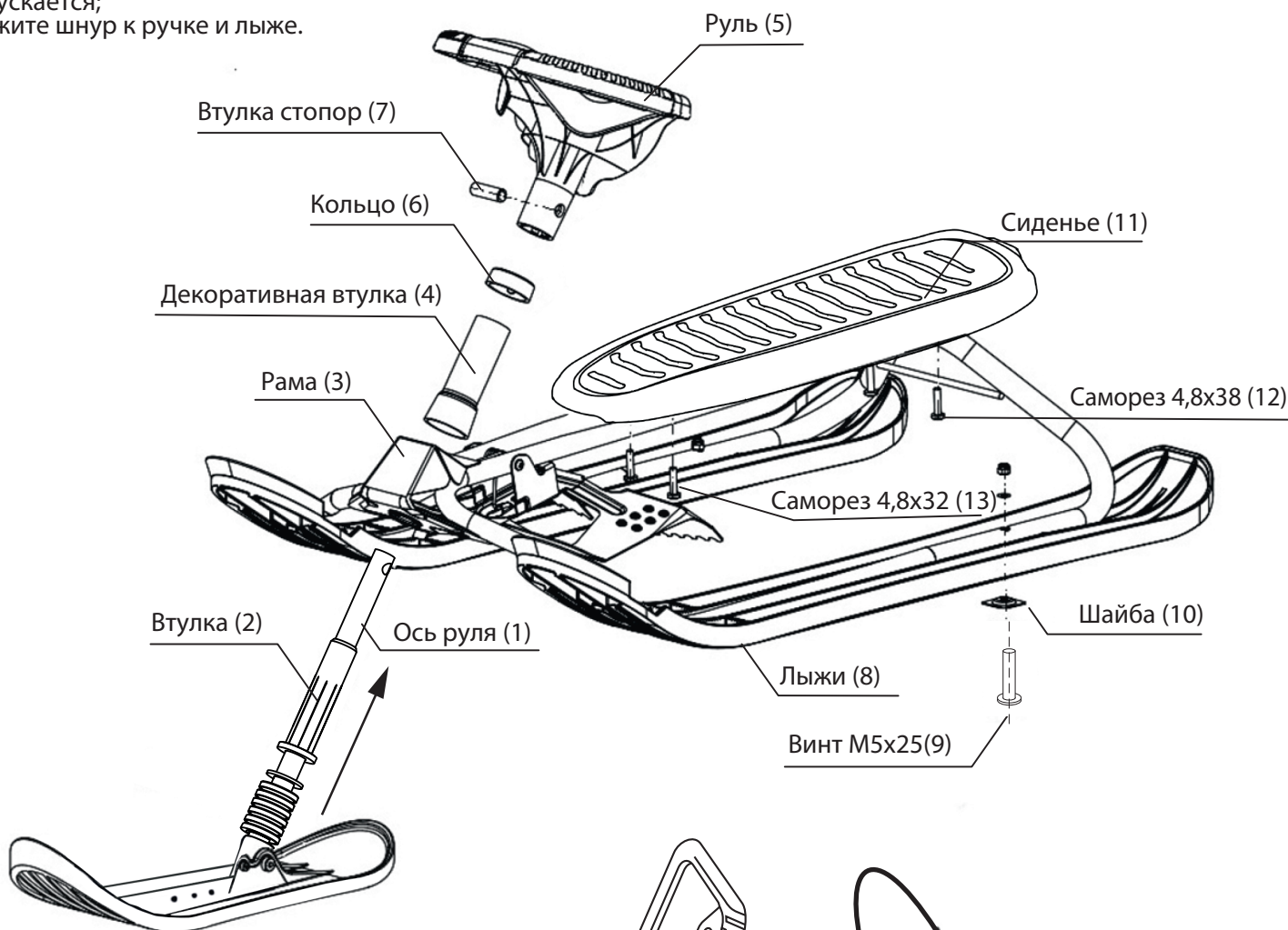
Рис.1 Сборка снегоката арт. ТСП
