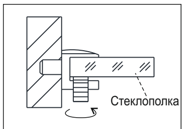
Полкодержатель П-образный
