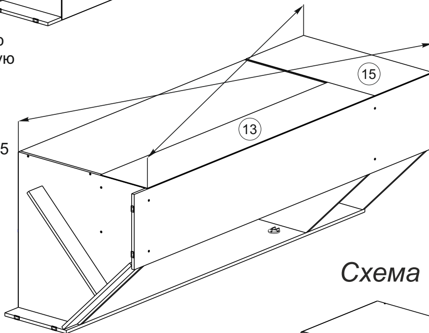
Монтаж толкателя
