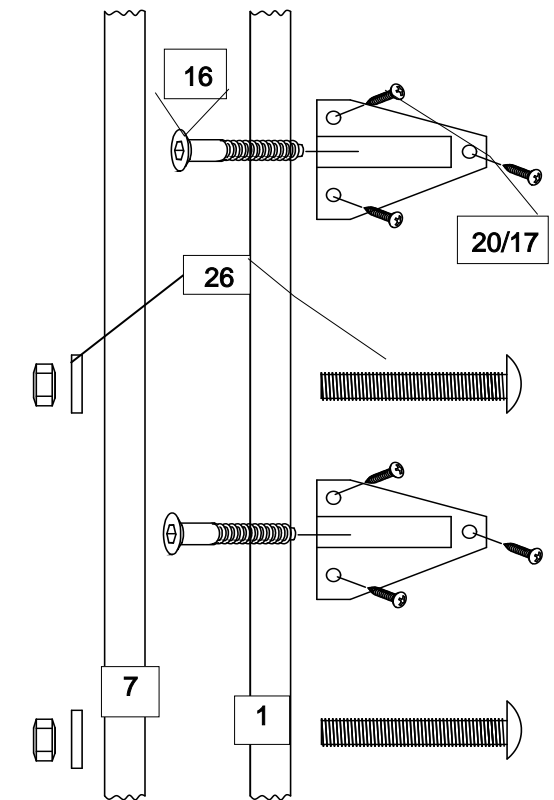
РИС.№1 (ВИД СЗАДИ)
