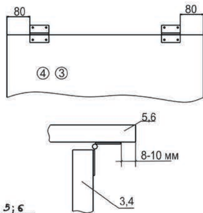
Рис.5 Крепление карточных петель.
