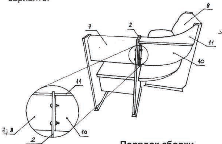
Порядок сборки.
